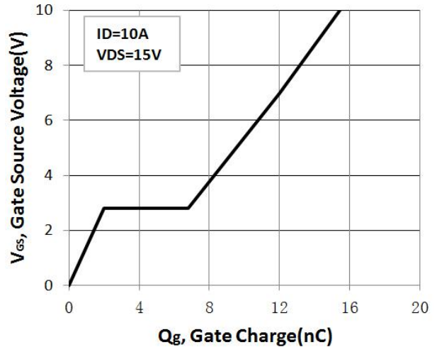
图 4 栅电荷波形
