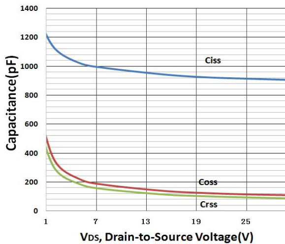
图 5 电容曲线
